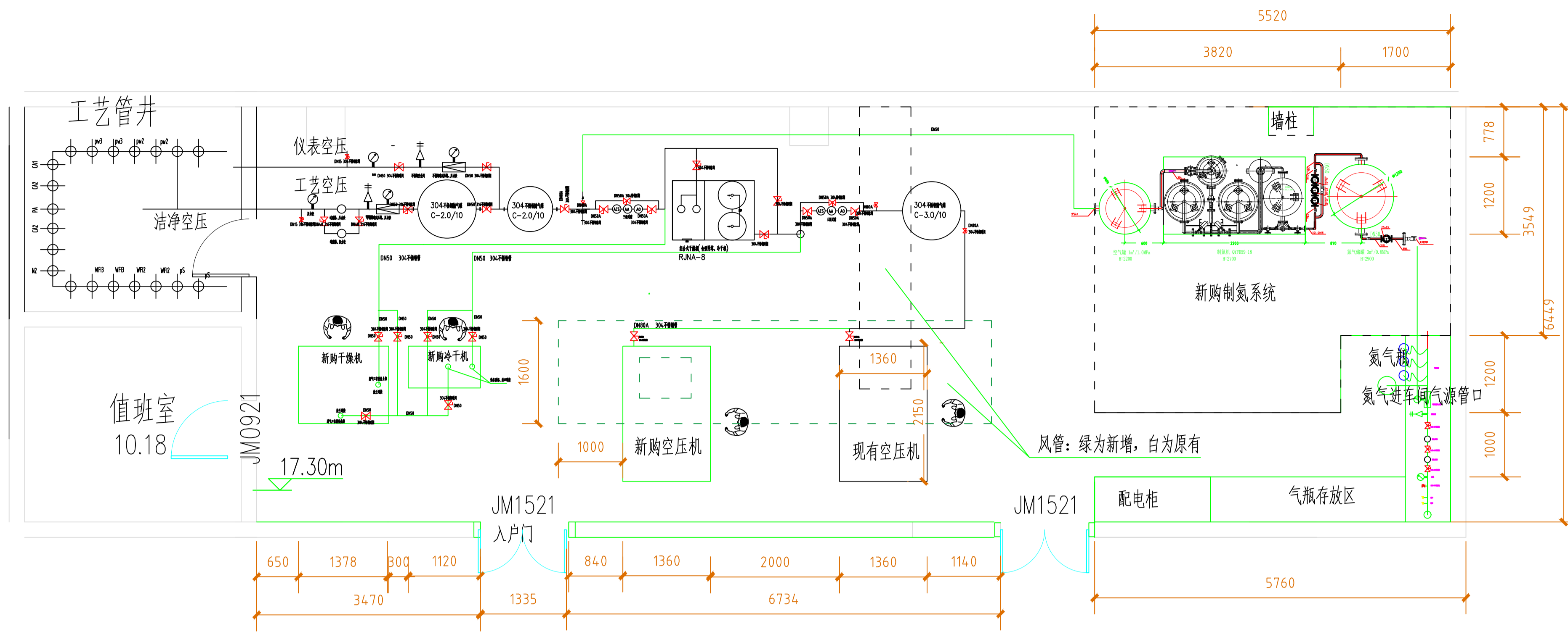
2022.1.28实测空压机房间尺寸图--新购空压机及制氮机平面布置图
